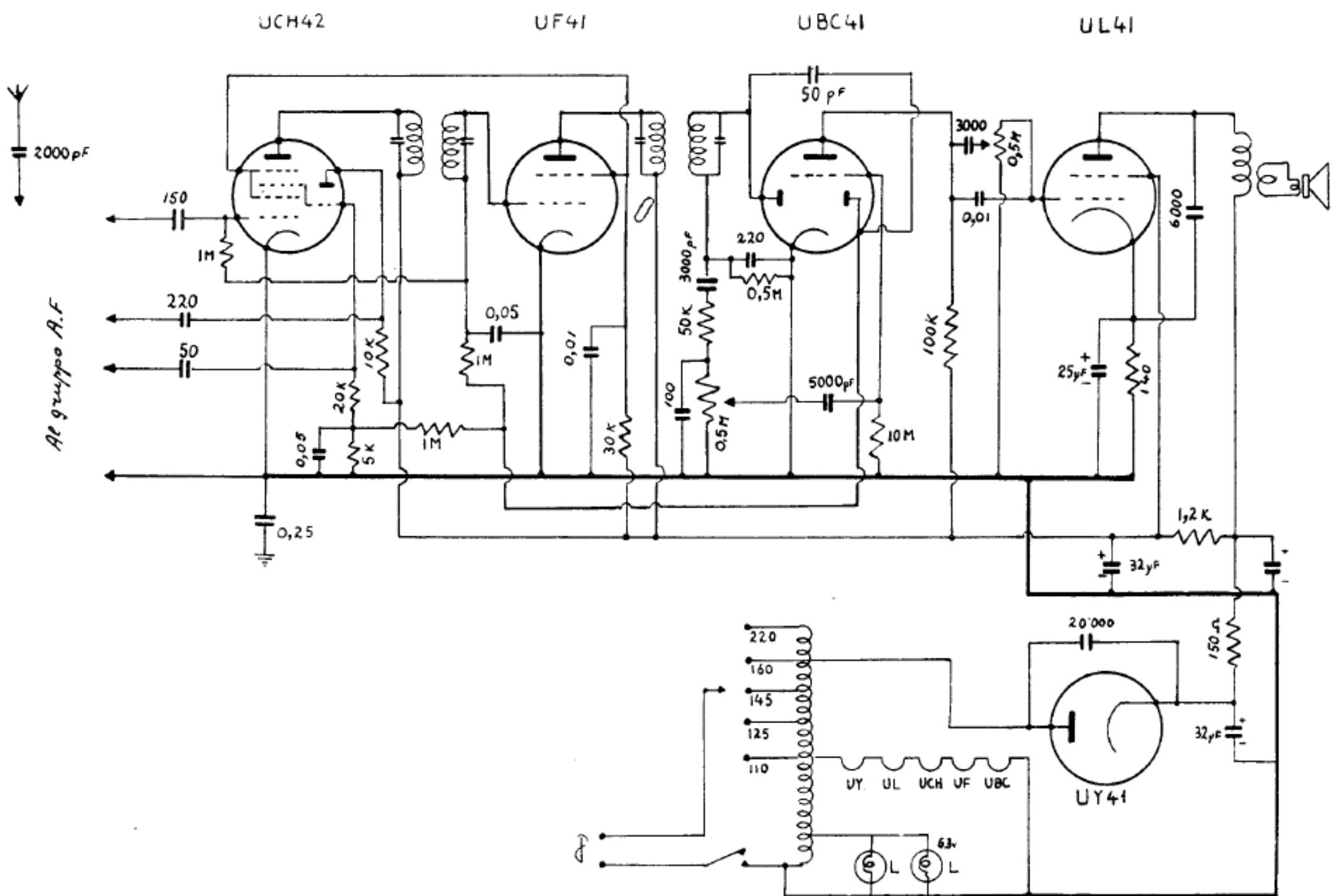
ALTAR - Mod. MR22. Lunghezza d'onda in metri: 12-26; 26-52; 180-580. Media frequenza 467 kc/s. Tensione al 1° elettrolitico 160 volt, al 2° 135 volt. Potenza d'uscita 3 watt.
